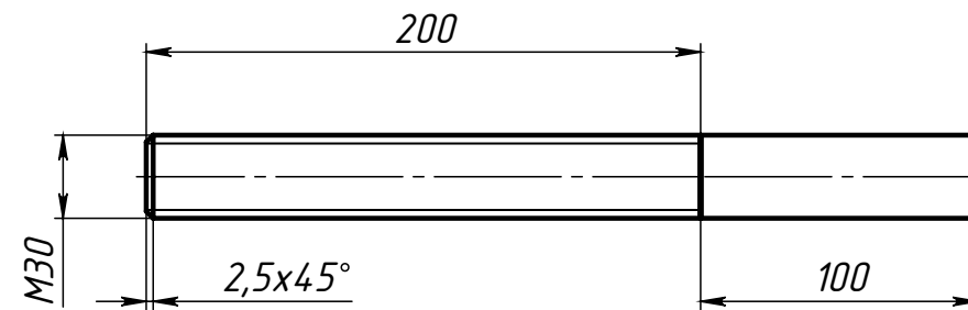
Поз.4 и Поз.8 (Шпильки резьбовые)
