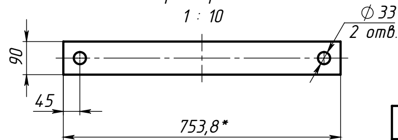
Поз.10 (Полухомут) развертка
