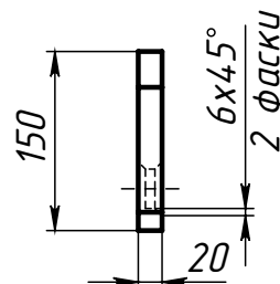
Поз.9 (Серьга)
