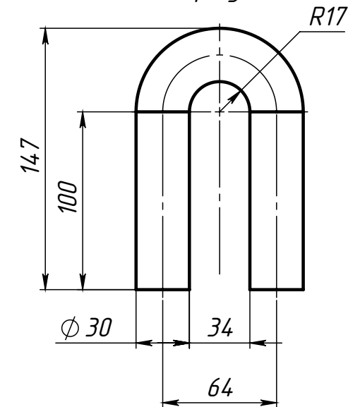
Поз.2 (Ушко)
