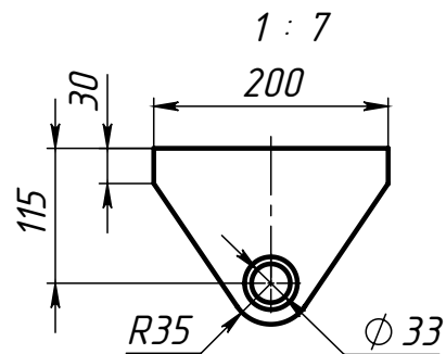
Поз.1 (Проушина)
